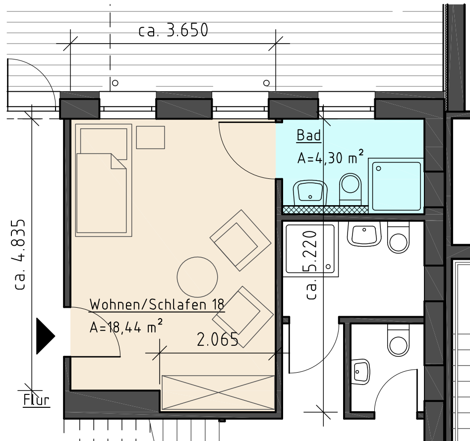
OG-Grundriss (Wohnung 18)
