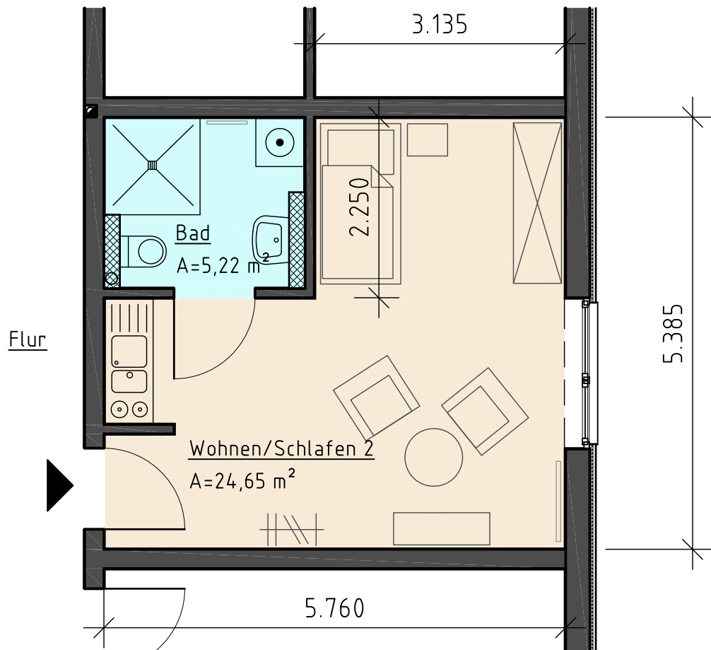
EG-Grundriss (Wohnung 2)
