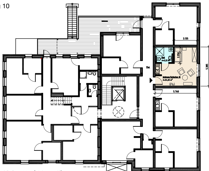
OG-Grundriss (Wohnung 10)
