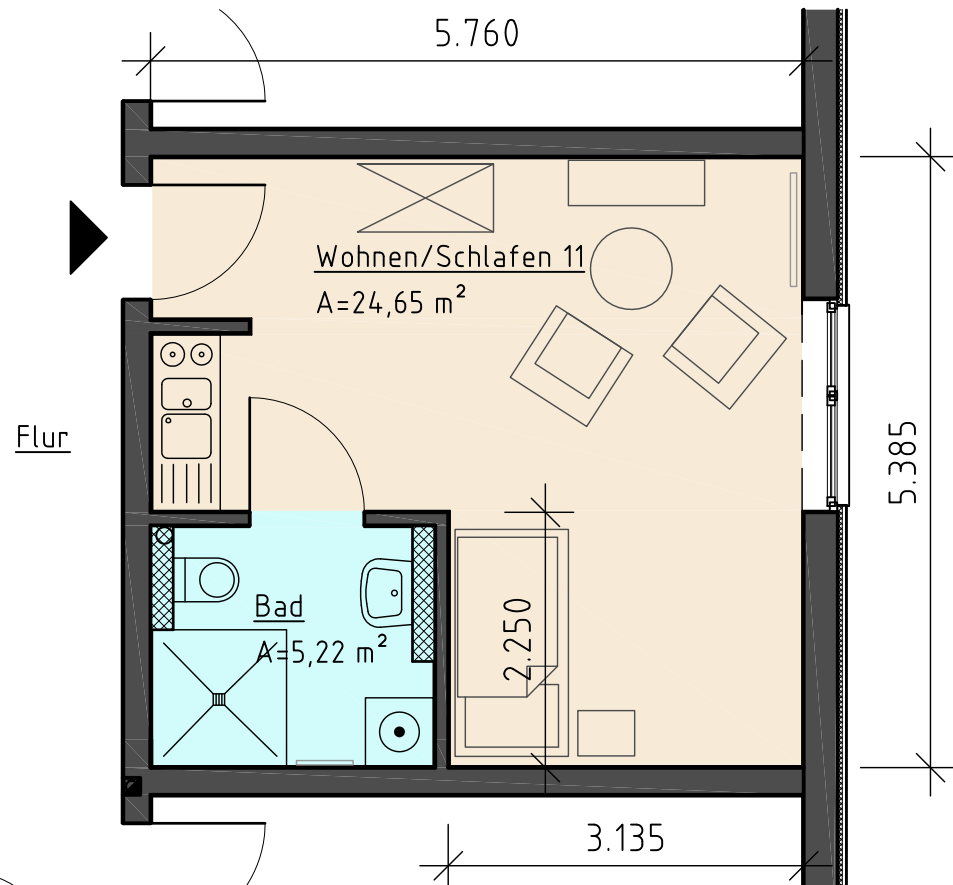
OG-Grundriss (Wohnung 11)
