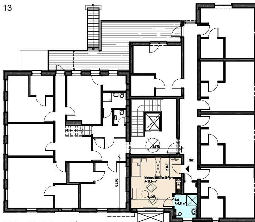
OG-Grundriss Wohnung 13)
