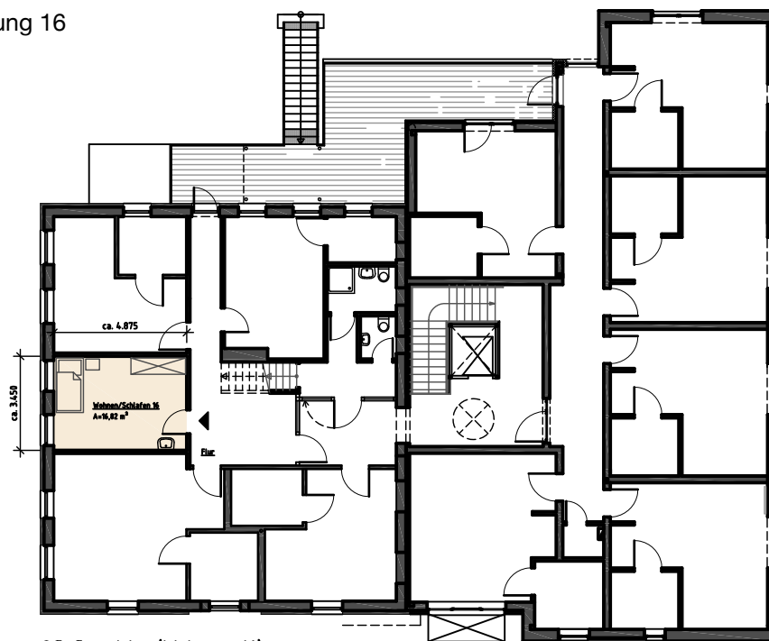
OG-Grundriss (Wohnung 16)
