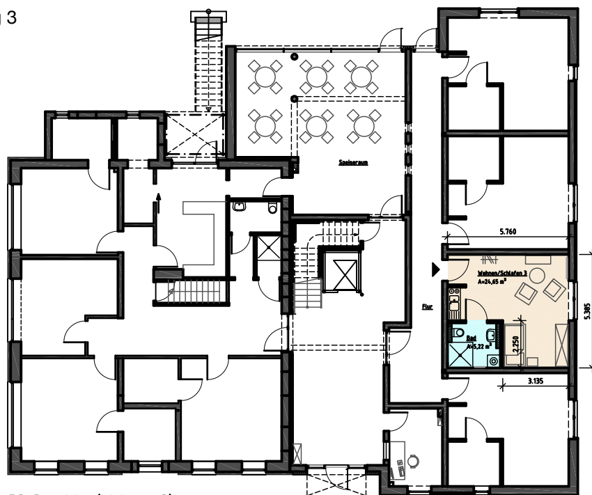
EG-Grundriss (Wohnung 3)
