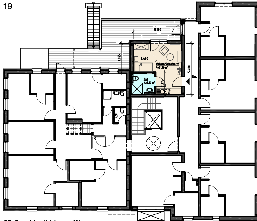
OG-Grundriss (Wohnung 19)
