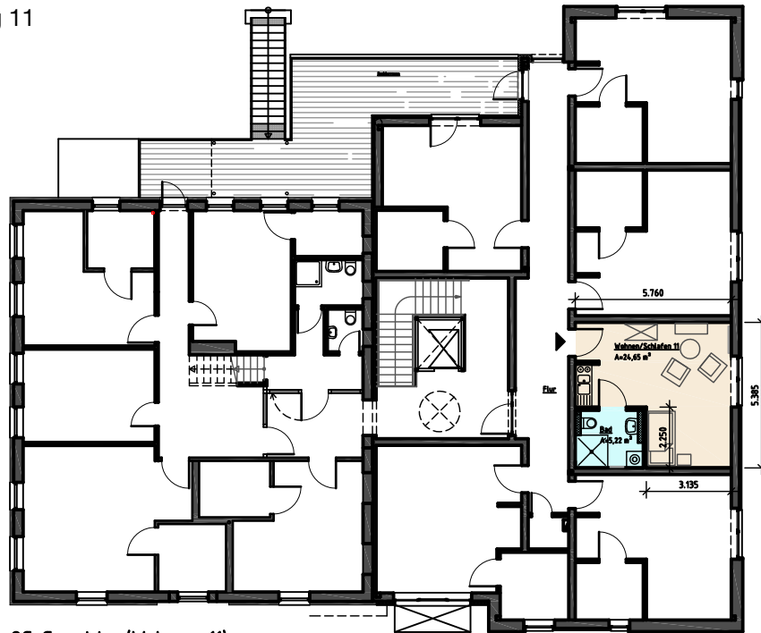
OG-Grundriss (Wohnung 11)
