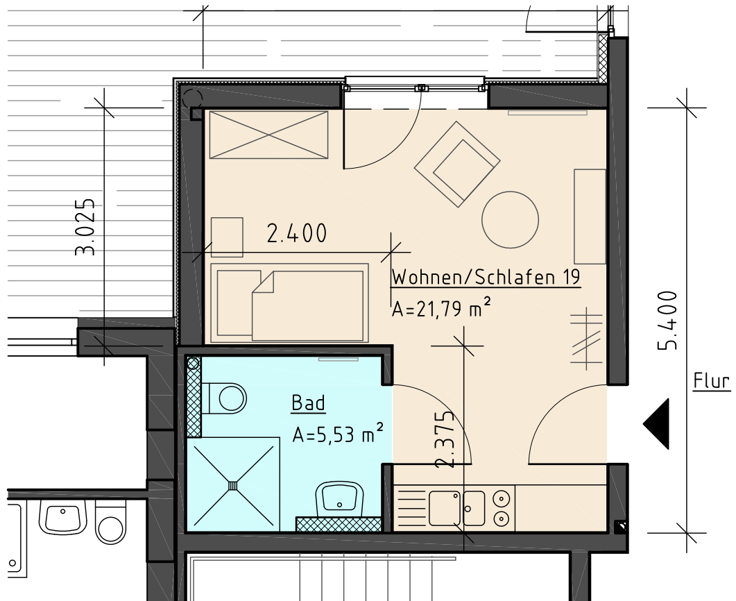
OG-Grundriss (Wohnung 19)
