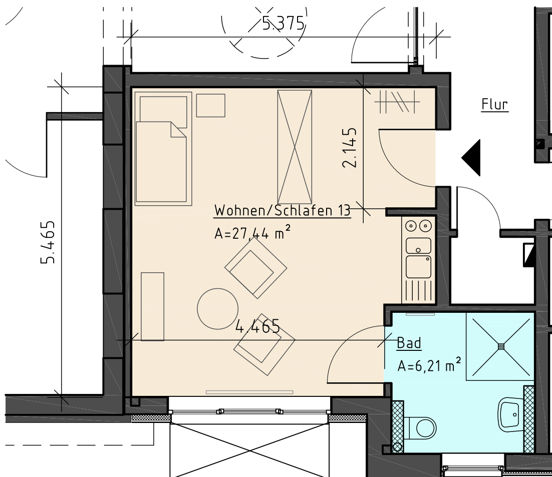
OG-Grundriss Wohnung 13)
