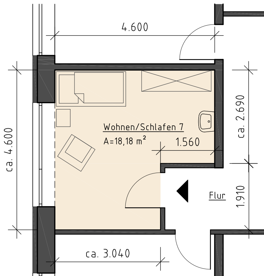
EG-Grundriss (Wohnung 7)
