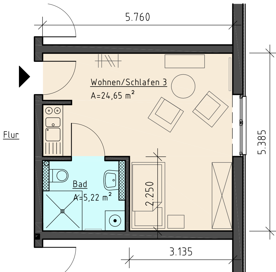
EG-Grundriss (Wohnung 3)
