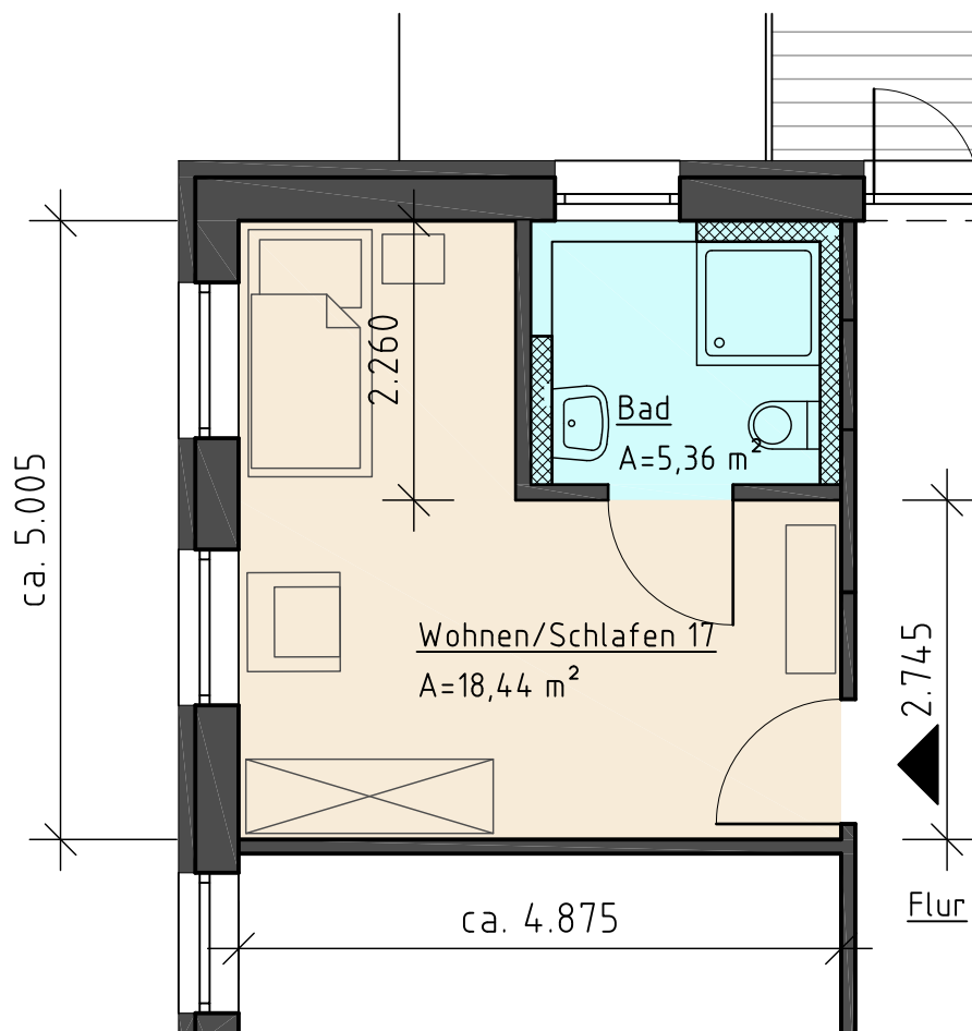
OG-Grundriss (Wohnung 17)
