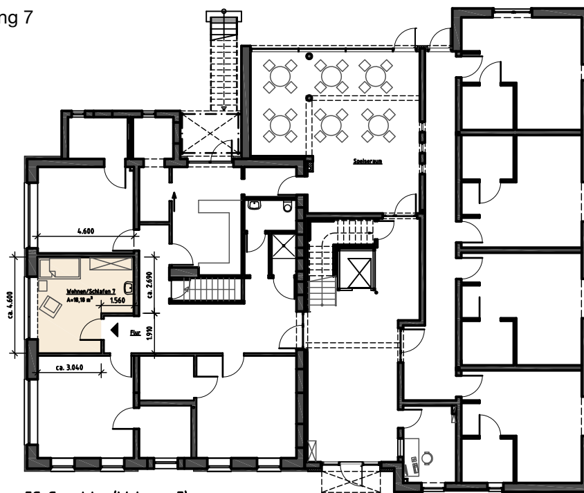
EG-Grundriss (Wohnung 7)
