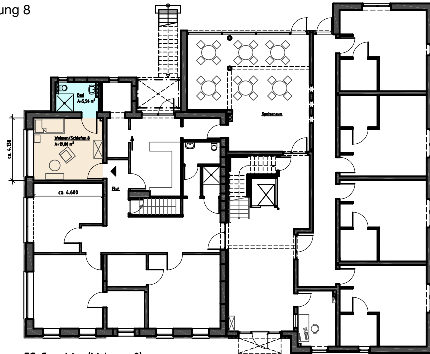
EG-Grundriss (Wohnung 8)
