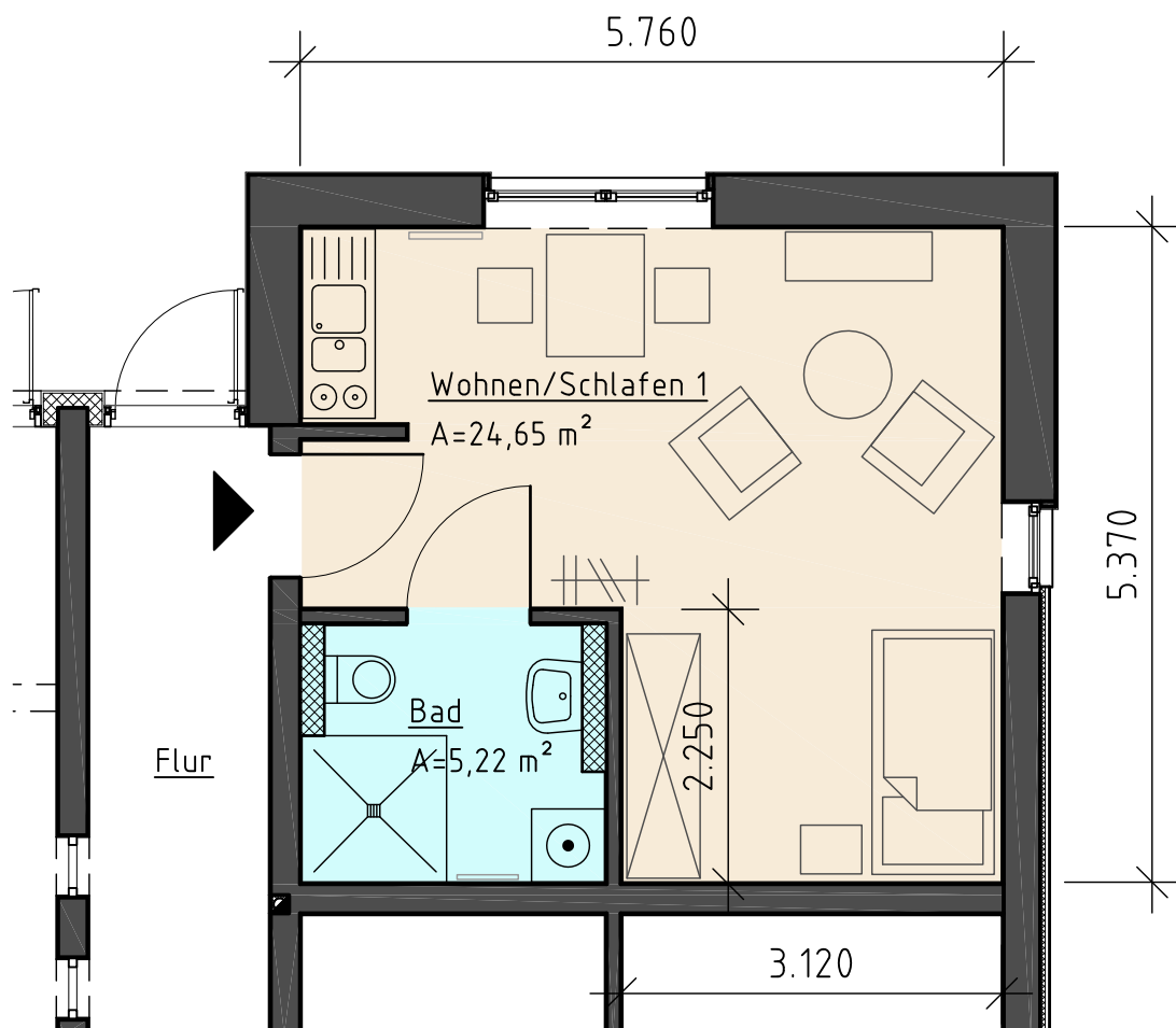
EG-Grundriss (Wohnung 1)
