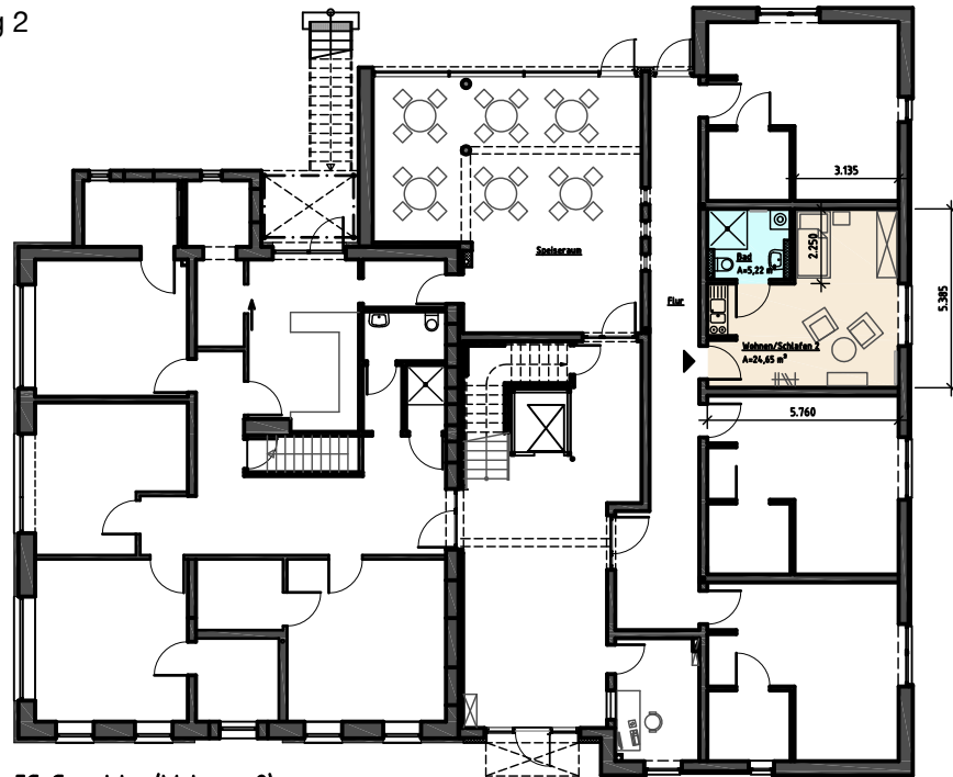
EG-Grundriss (Wohnung 2)
