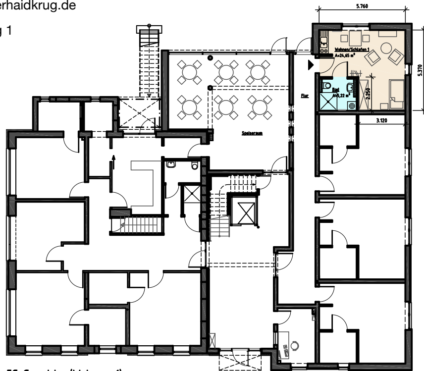
EG-Grundriss (Wohnung 1)
