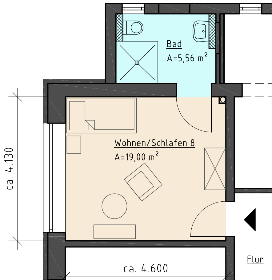
EG-Grundriss (Wohnung 8)
