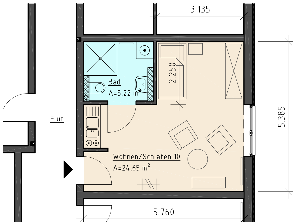
OG-Grundriss (Wohnung 10)
